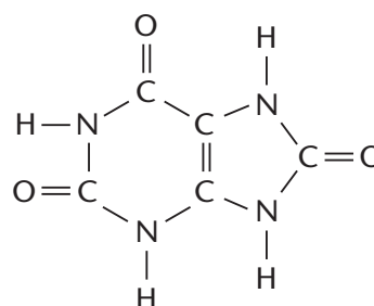
Ácido úrico
