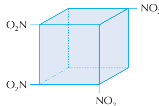
Tetranitrocubano
