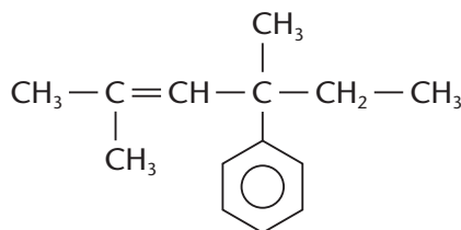
4-fenil-2,4-dimetil-hex-2-eno
