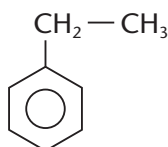
Etil-benzeno
