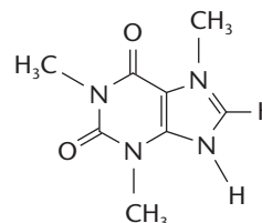
Cafeína
