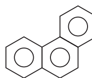
Fenantreno
