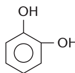
Difenol
