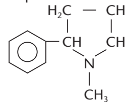
Nicotina
