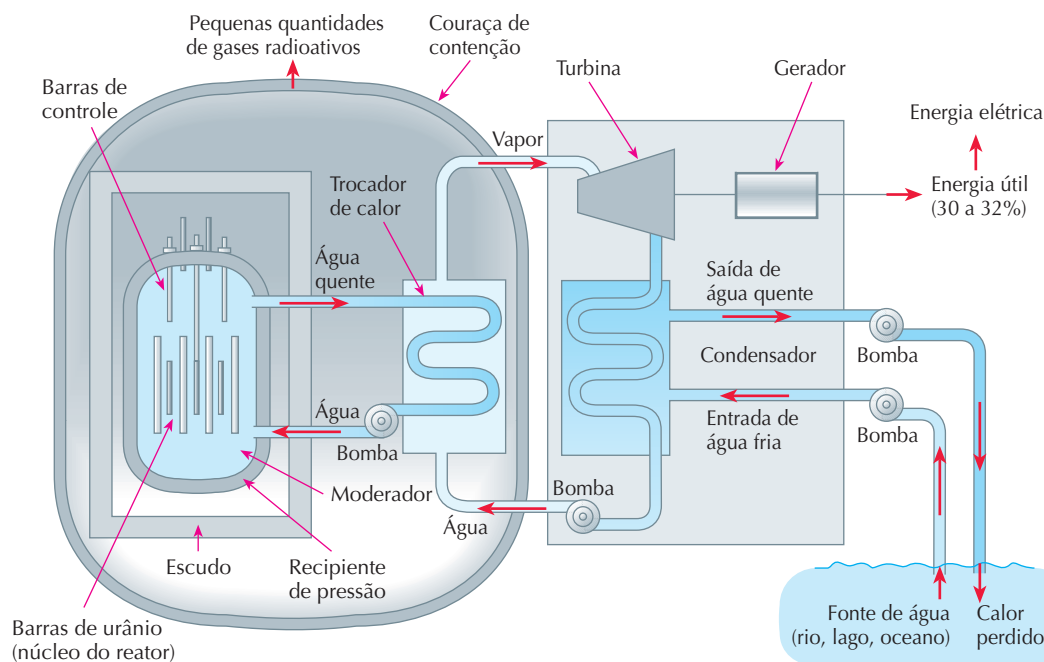
Esquema de um reator nuclear de água pressurizada (PWR, pressurized water reactor ) semelhante ao usado na Usina de Angra dos Reis.
